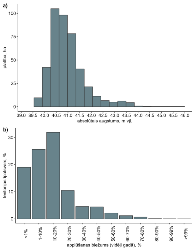
1.3.4.7. att. a) DL “Burtnieka ezera pļavas” teritorijas absolūto augstumu sadalījums; b) DL “Burtnieka ezera pļavas” teritorijas applūšanas biežums (balstoties uz ikgadējo ūdens līmeņa ilguma līkni).
