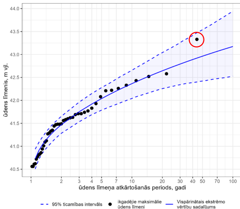
1.3.4.5. att. Plūdu atkārošanās biežuma modelis Burtņieka maksimālajiem ūdens līmeņiem (ar sarkanu apvilktu 1956. gada augstākais ūdens līmenis)
