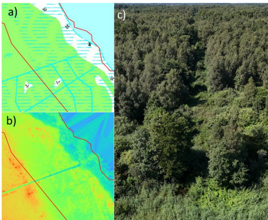
1.3.4.15. att. Nereģistrēts meliorācijas grāvis DLteritorijā starp Grausta sēri un Ataku. Topogrāfiskajā kartē (a, LĢIA) attēloti vairāki grāvji, no kuriem viens ir identificējams DRM (b attēls). Skats uz grāvi dabā no ezera puses uz R (c).
