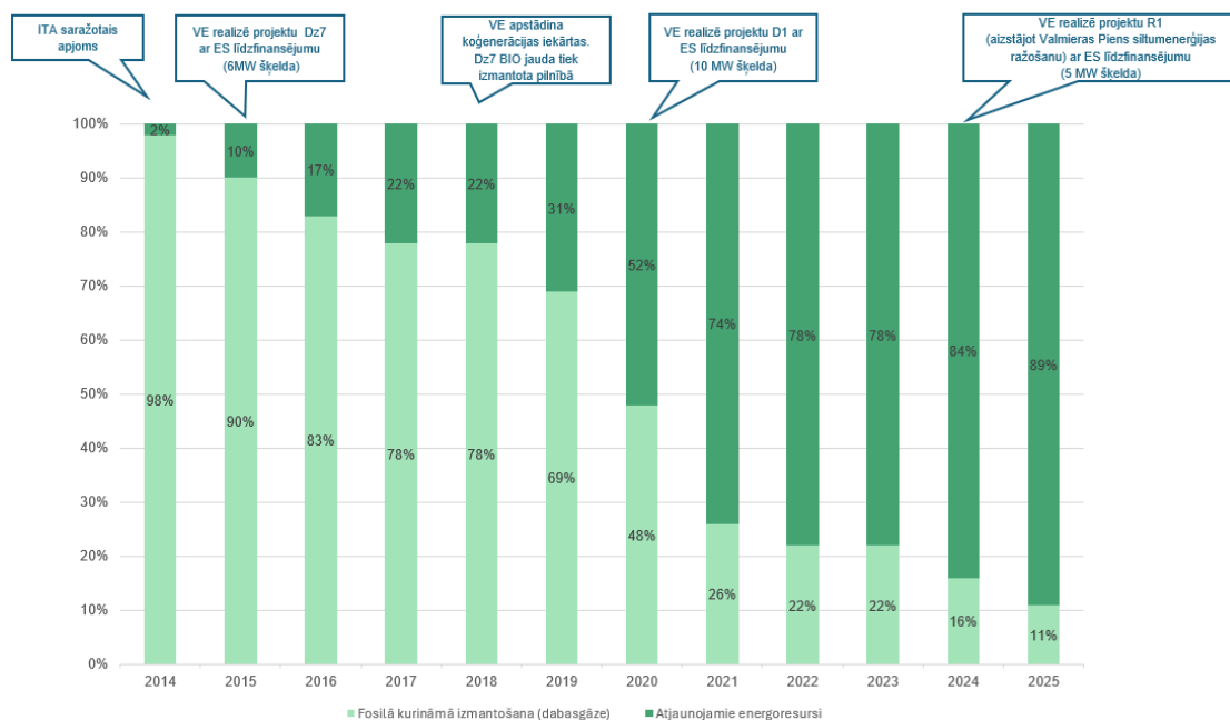
7. grafiks. Valmieras pilsētas centralizētajā siltumapgādē izmantotā kurināmā balance. Avots: AS "Valmieras Enerģija".
