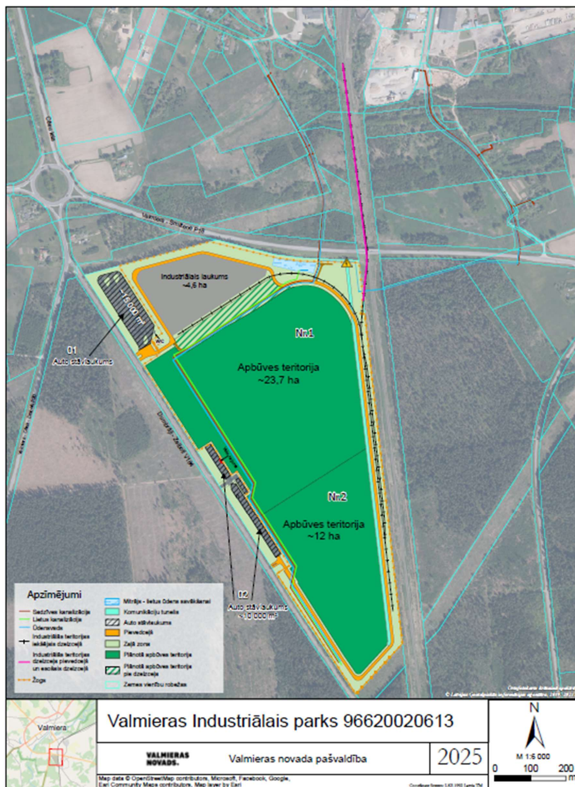
Valmieras Industriālā parka teritorijas plānojums
