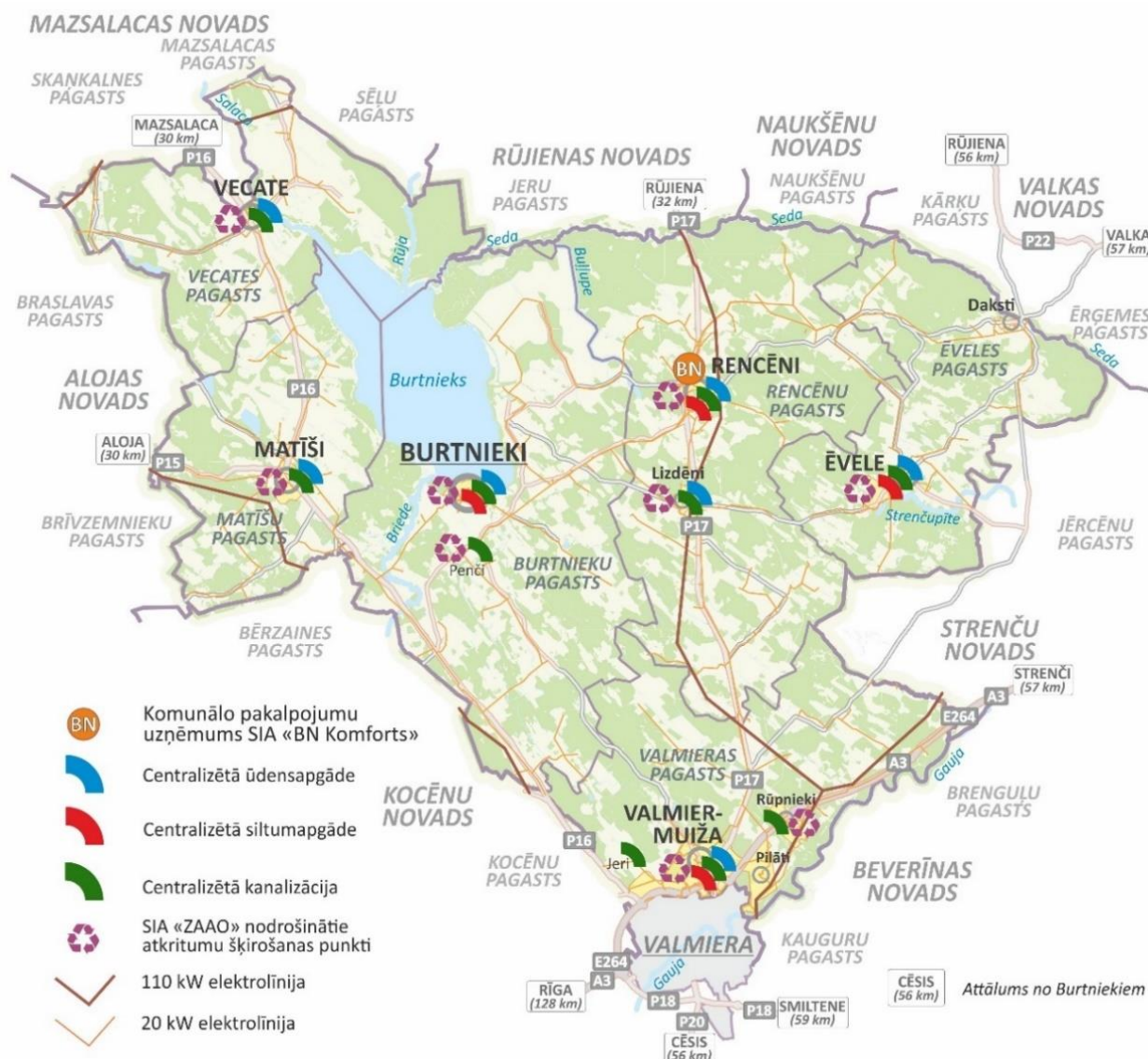
ATTĒLS:79. INŽENIERTEHNISKĀ INFRASTRUKTŪRA BURTNIIEKU NOVADĀ
