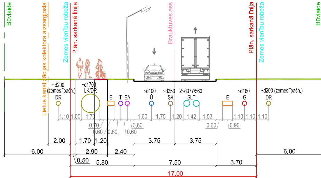
Šķēršprofils 1-1, variants C (plānotais Dakstiņu ielas posms)
