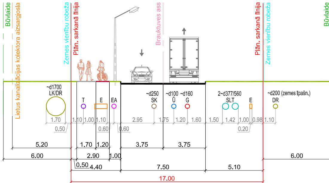
Šķēršprofils 1-1, variants B (plānotais Dakstiņu ielas posms)
