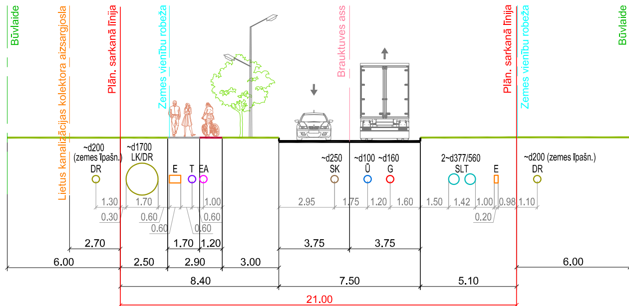
Šķēršprofils 1-1, variants E (plānotais Dakstiņu ielas posms)
