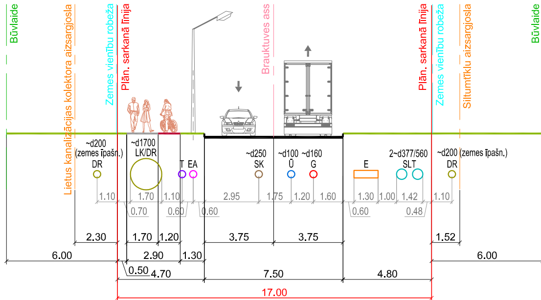
Šķēršprofils 1-1, variants A (plānotais Dakstiņu ielas posms)
