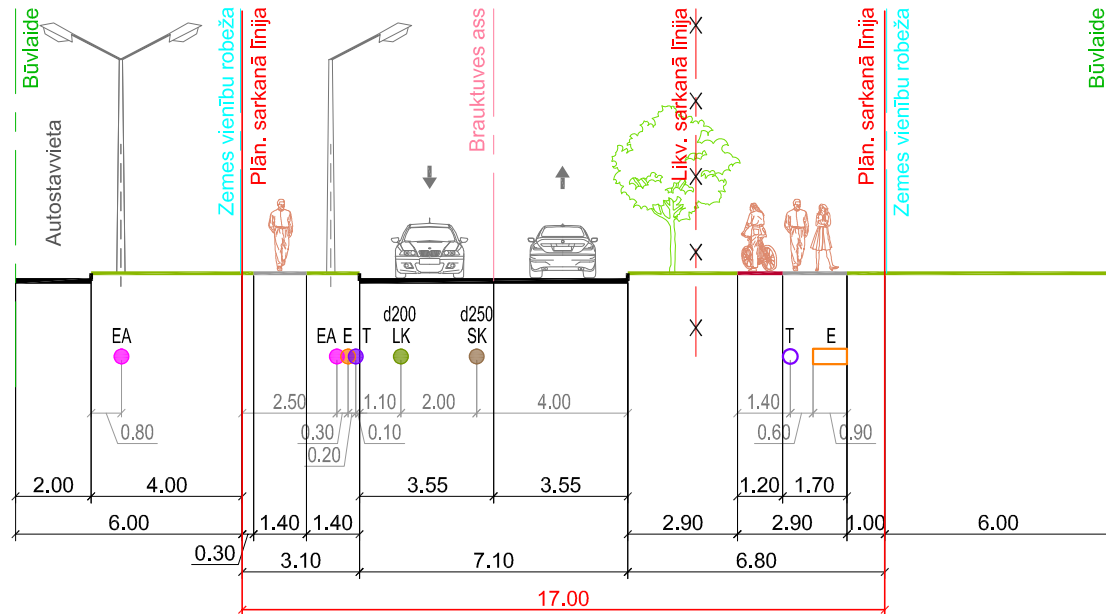
Šķēršprofils 2-2 (esošais Ķieģeļu ielas posms)
