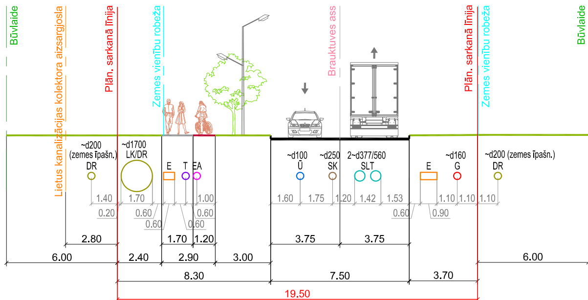
Šķēršprofils 1-1, variants D (plānotais Dakstiņu ielas posms)
