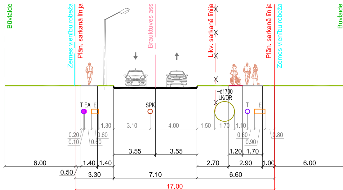
Šķēršprofils 3-3 (plānotais Ķieģeļu ielas posms)
